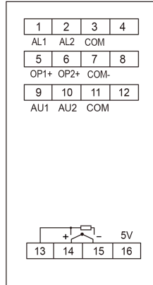
新 D71 接线图
